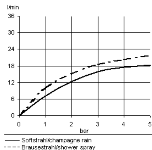
Diagram przepływu
